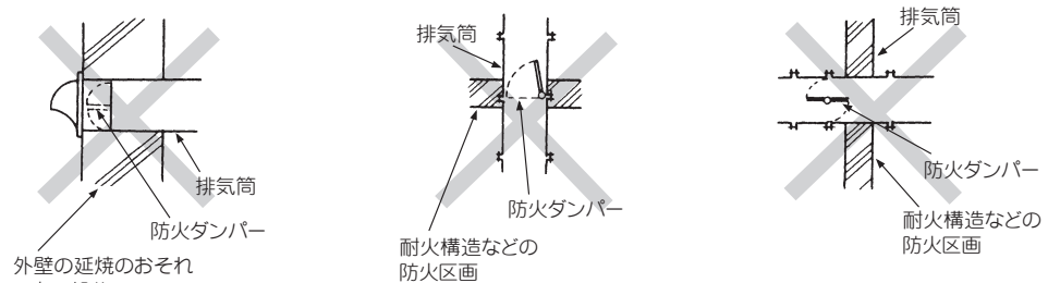
図-15 防火ダンパー取り付け禁止の例
