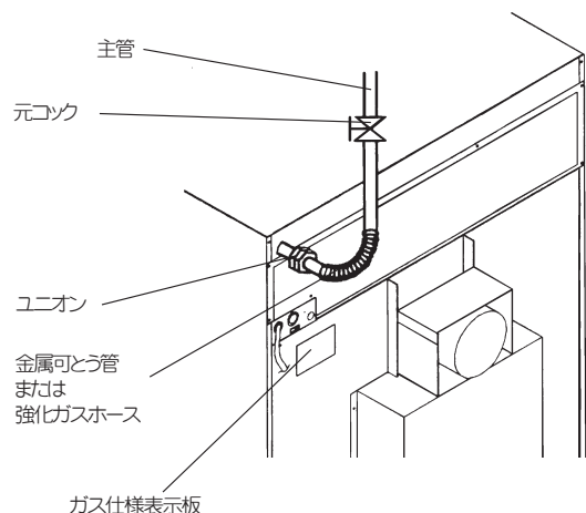
図-13 ガス配管
