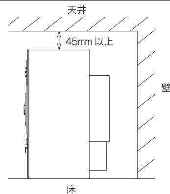
図 -11 設置側面図
