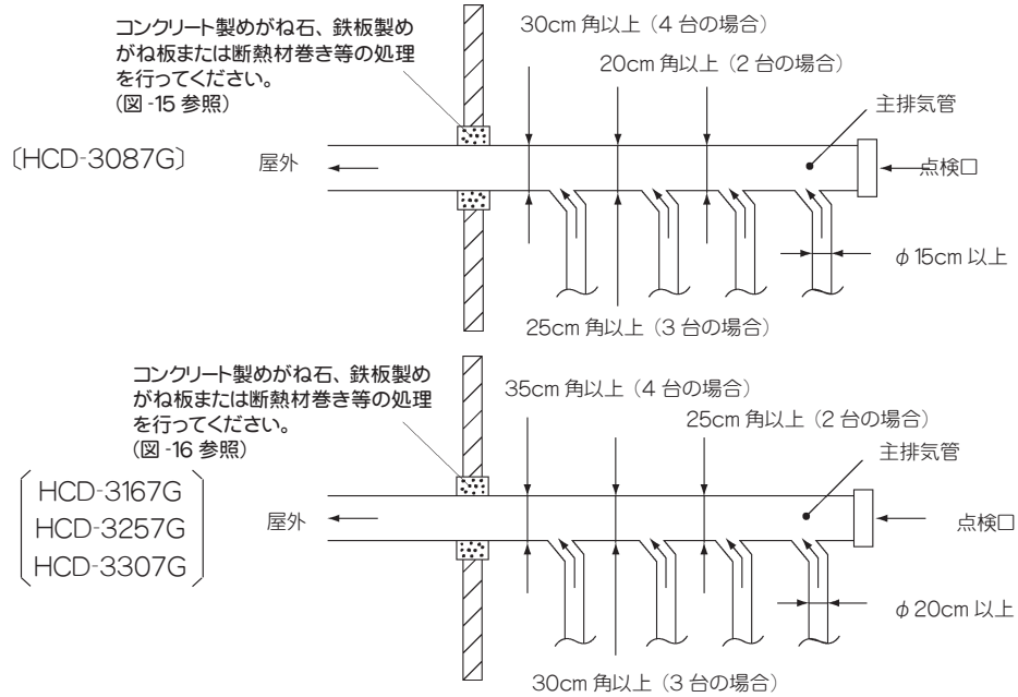
図-14 集合ダクト
