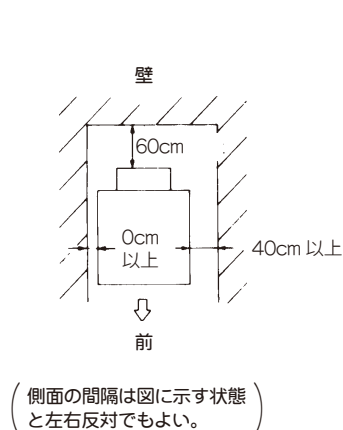
図-9 設置平面図
