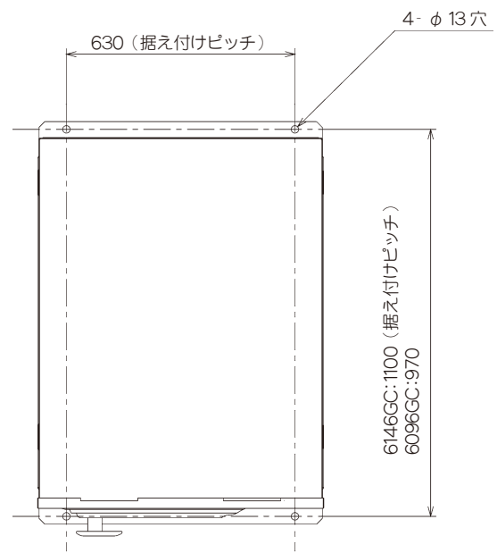
図 - 13 据え付けピッチ
