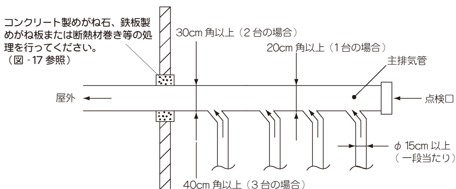
図-15 集合ダクト
