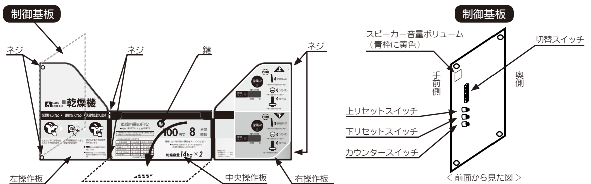
図-22 操作板と制御基板
