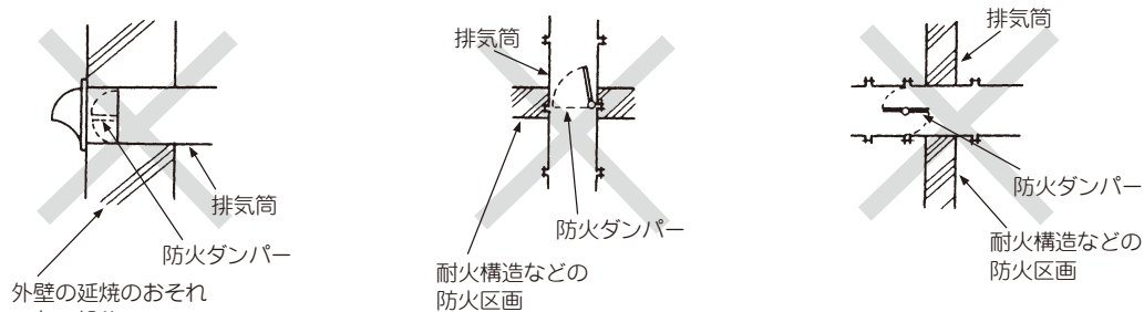
図-16 防火ダンパー取り付け禁止の例
