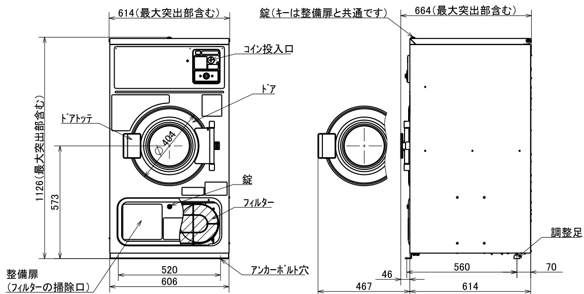
(側面図)
