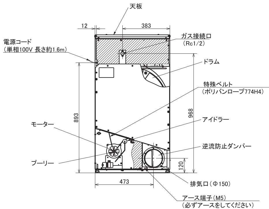
(背面図)
