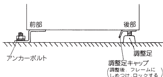
図ー 12 アンカー穴、調整足位置
