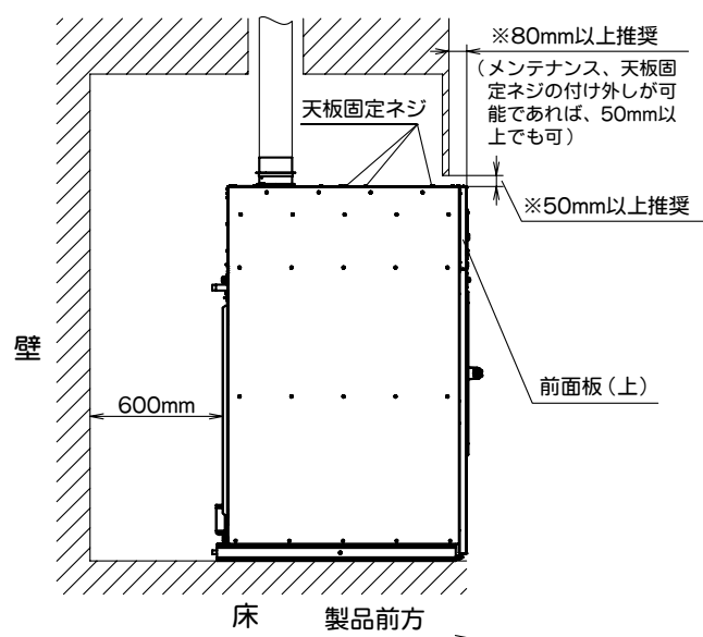
図7 設置側面図
