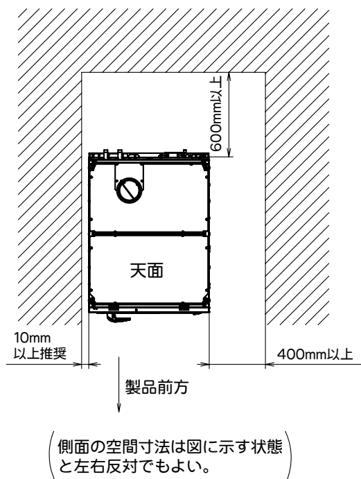
図6 設置平面図
