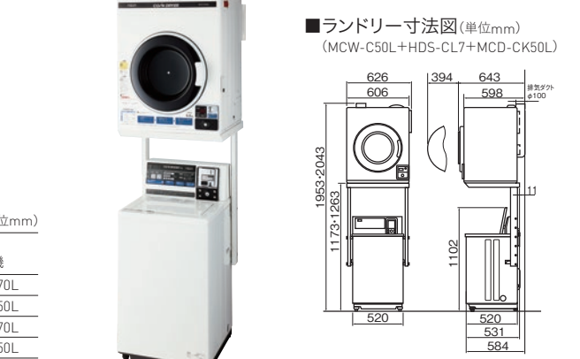
■ランドリー寸法図(単位:mm)(MCW-C50L+HDS-CL7+MCD-CK50L)
