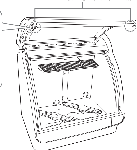
ドアフック取り付け位置(2カ所)
