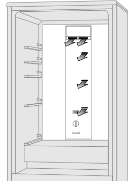
冷蔵室冷気吹出口図
