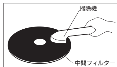
中間フィルターの掃除
