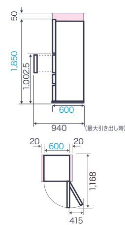
■据付必要寸法図(単位:mm)
