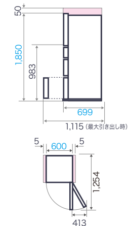
■据付必要寸法図 (単位: mm)
